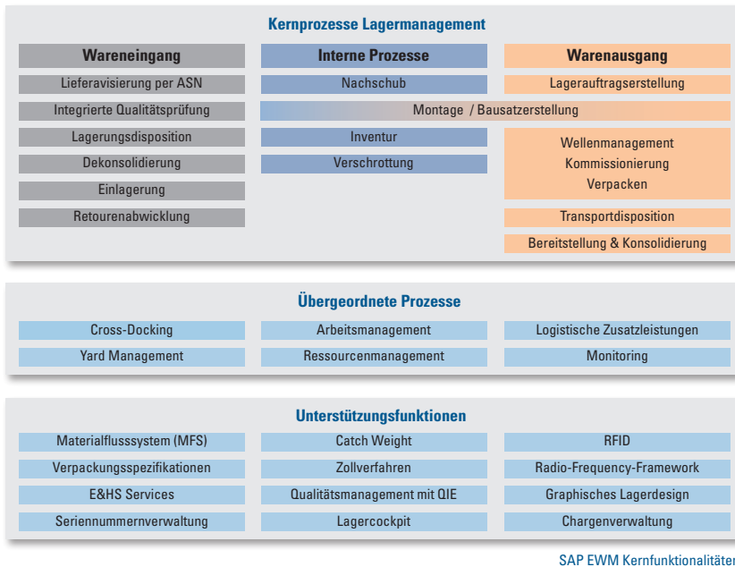
SAP EWM Kernfunktionalitäten
