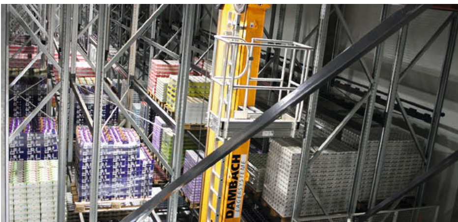
Das Regalbediengerät ist mit einer doppeltiefen Teleskopgabel ausgestattet
