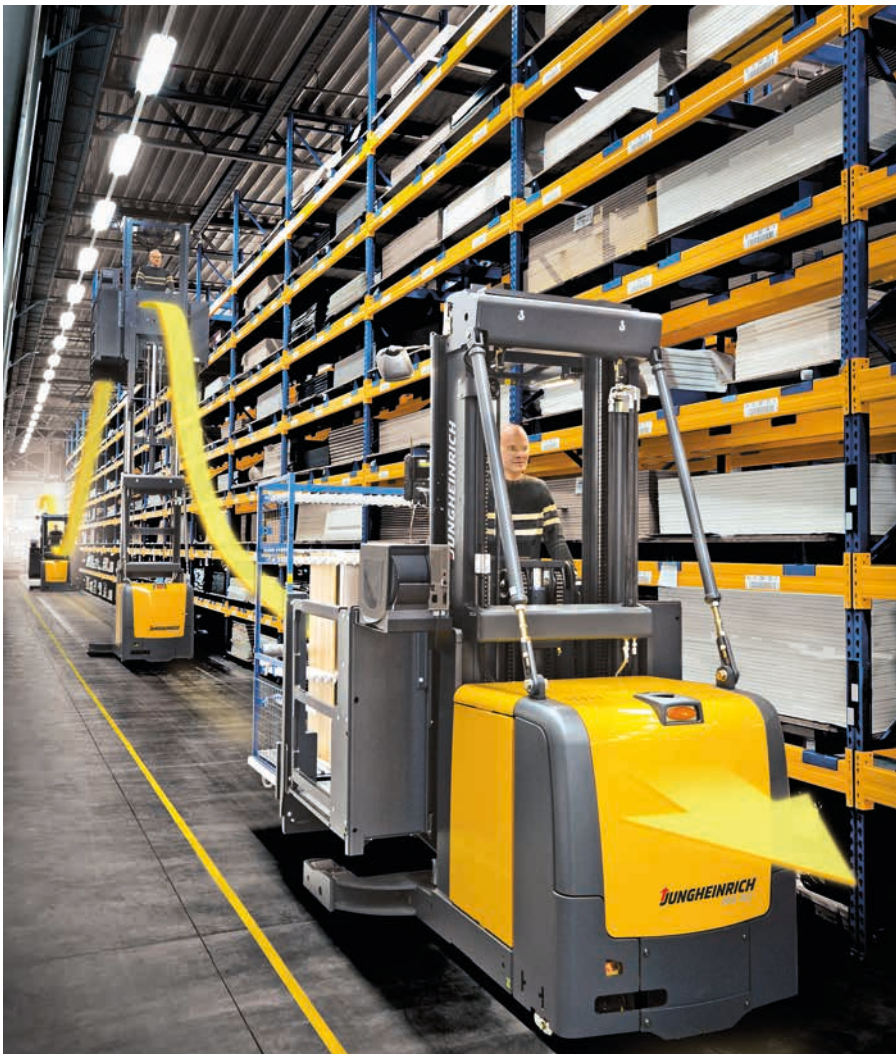
▲ Synchronisierter Material- und Informationsfluss im Schmalganglager: Halbautomatische Anfahrt der Positionen mit einem Vertikalkommissionierer EKS und Lagernavigation
