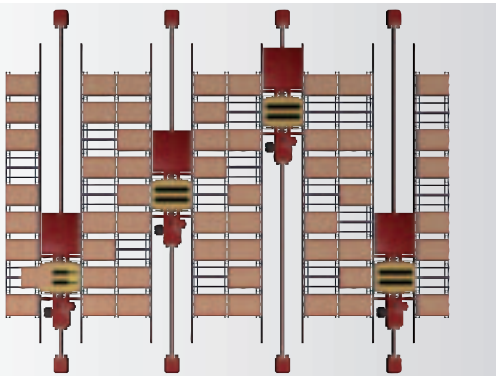
Einzelplatzlager
