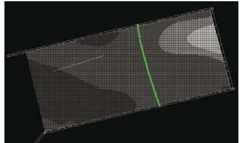
Abb. 2: Flözdraufsicht in PSImcontrol mit Verlauf der aktuellen Abbaufont (grüne Linie)
